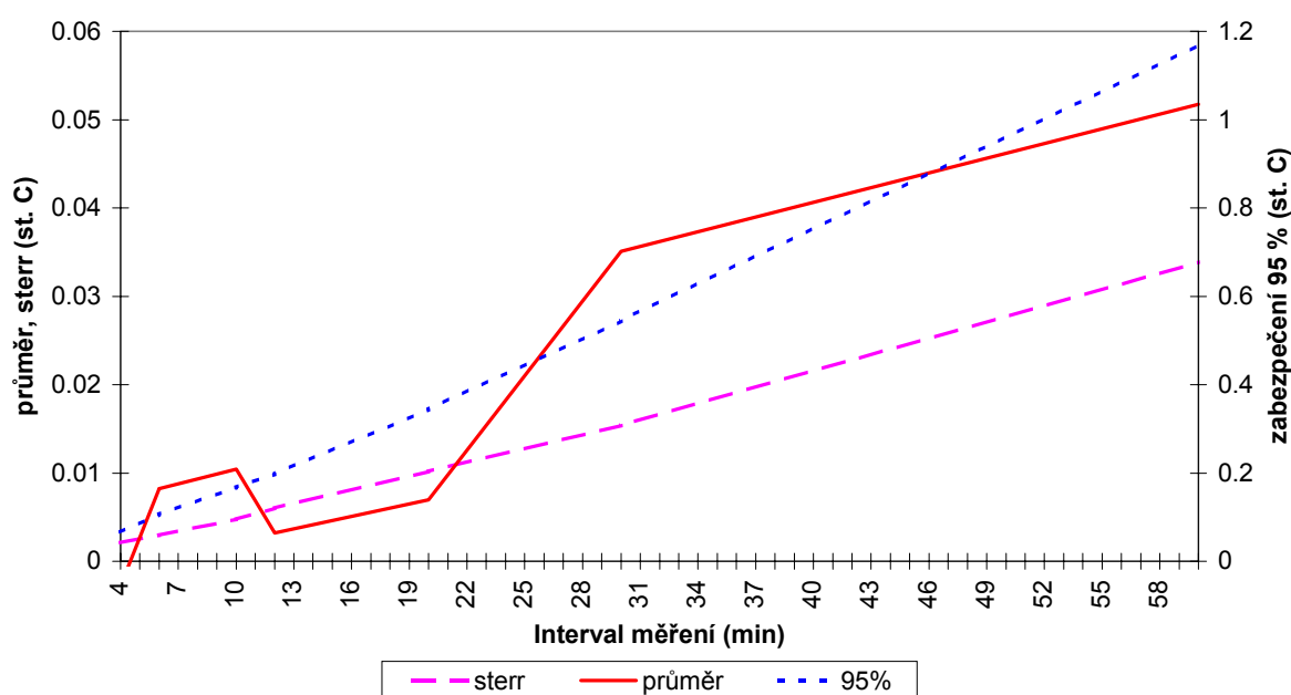
Průběh základních statistických charakteristik odchylek pro jednotlivé intervaly měření (hodinové průměry)
